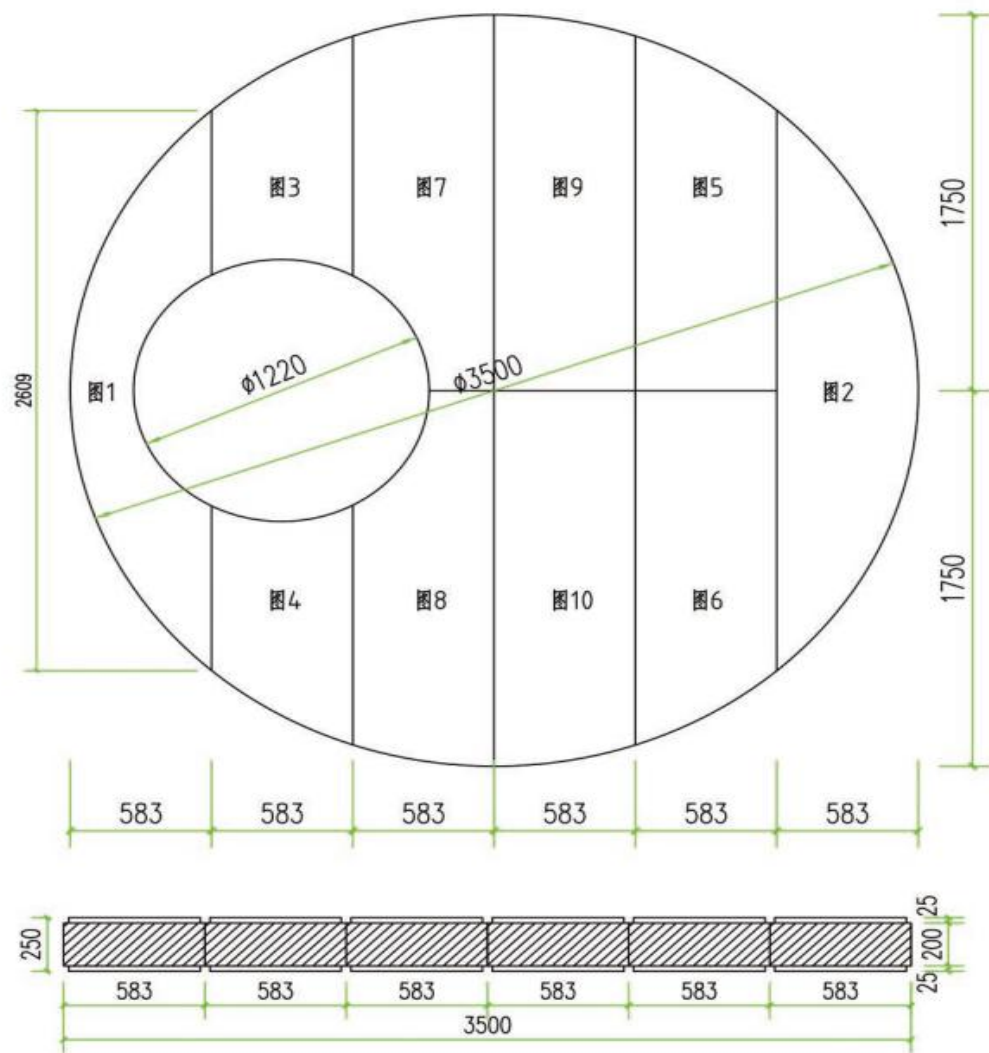
\phi 3500 分块示意图
