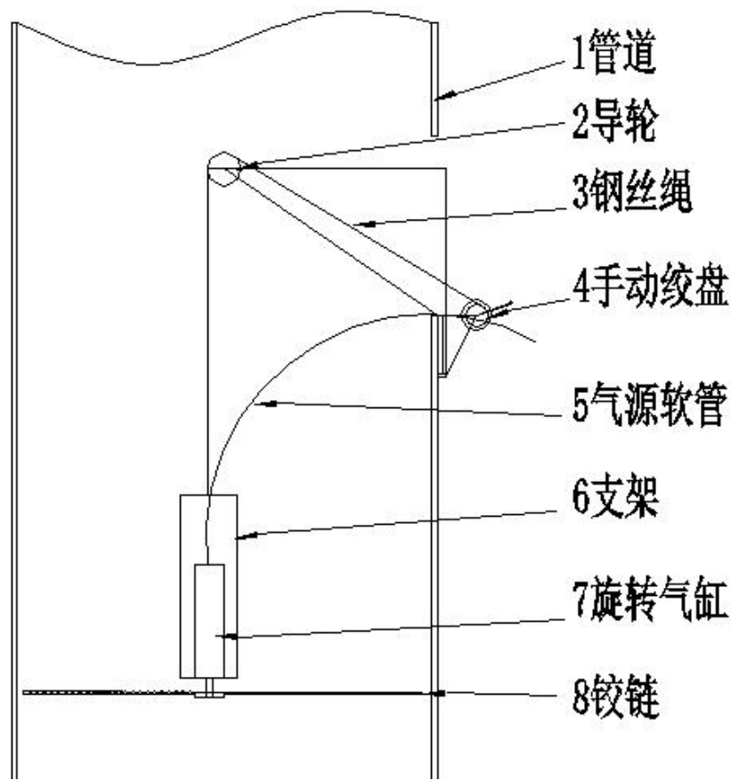
设备简图
