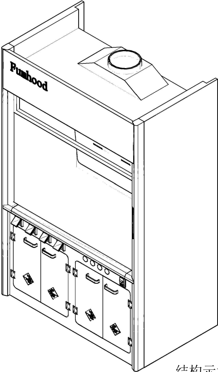
结构示意图
